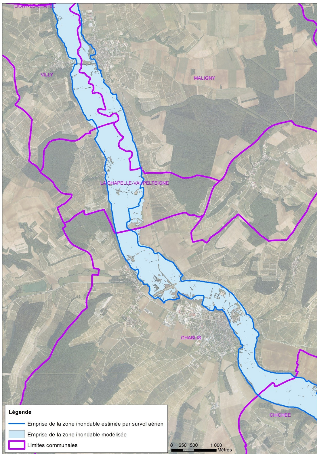
Figure 19 : Comparaison des emprises maximales d’inondation observées et simulées lors de la crue de mai 2013 entre Chablisy et Maligny
